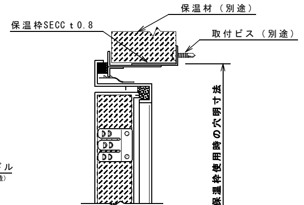
保温枠使用の場合 (ケーシングに外側保温をする場合)
