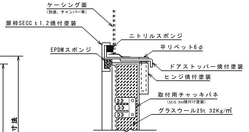
a部詳細
