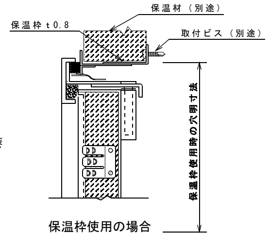
a部詳細
