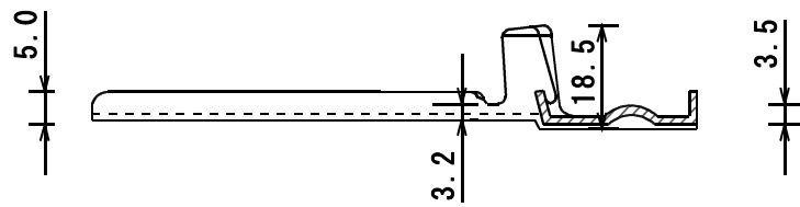
A-A 断面
