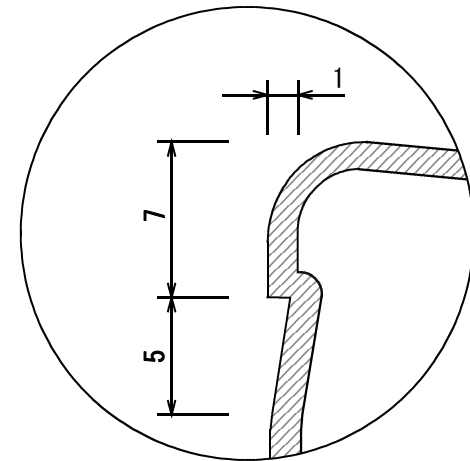
ストッパー詳細
