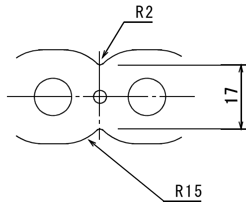
切欠き部詳細
