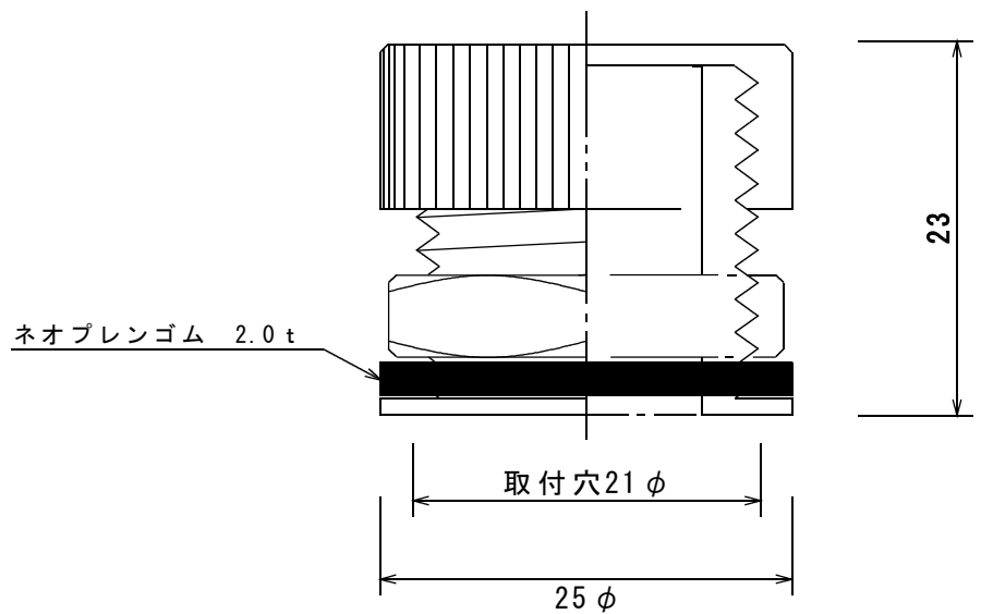
取付穴径21φ・全長23mm
