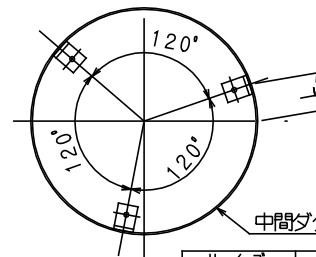
L金具取付要領図 (天井状図)
