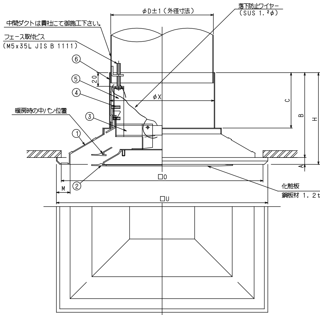
落下防止取付要領図
