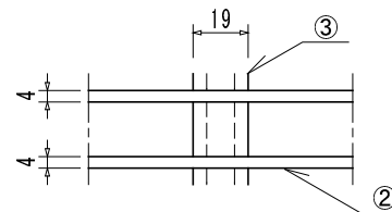
羽根補強要領 有効寸法h>800
