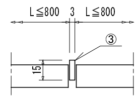
羽根分割要領 有効寸法h
