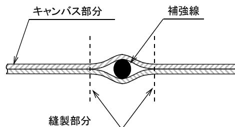
a部断面
